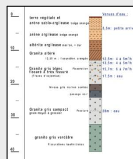
▲ Coupe géologique d'un des 6 forages réalisés
